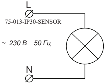
Рисунок 3. Схема подключения светильника 75-013-IP30-SENSOR
